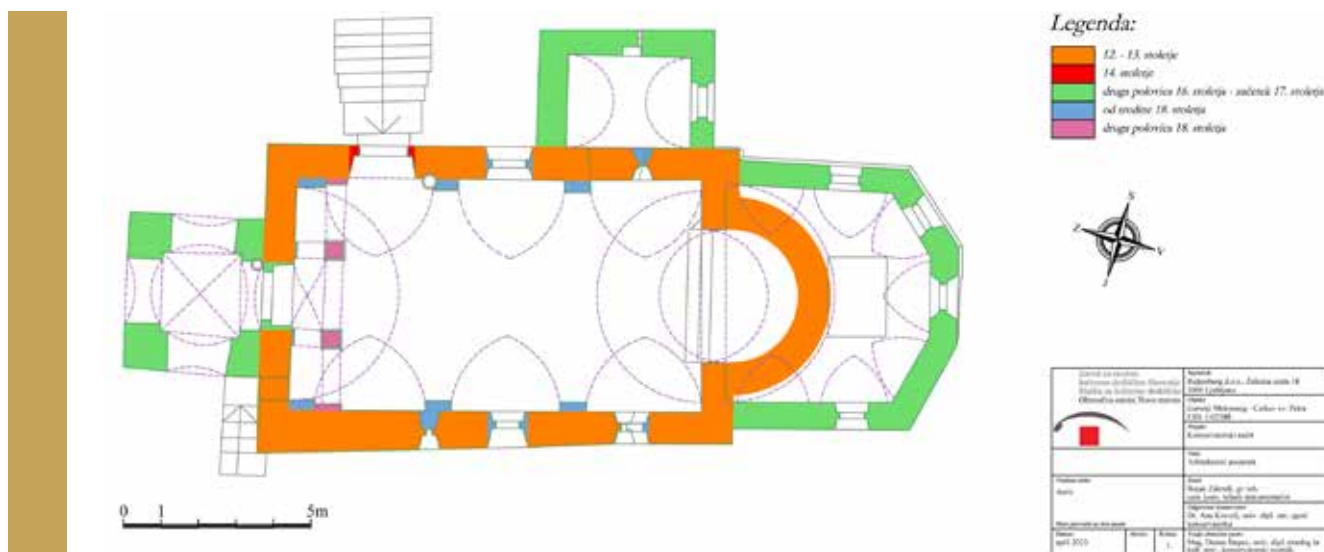
Slika 1: Tloris cerkve sv. Petra v Gorenjem Mokronogu, izdelal: Bojan Zaletelj.
