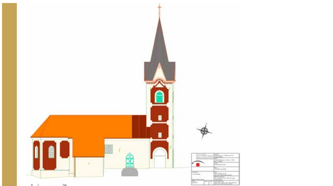
Slika 2: Severna fasada cerkve sv. Petra v Gorenjem Mokronogu, izdelal: Bojan Zaletelj.
