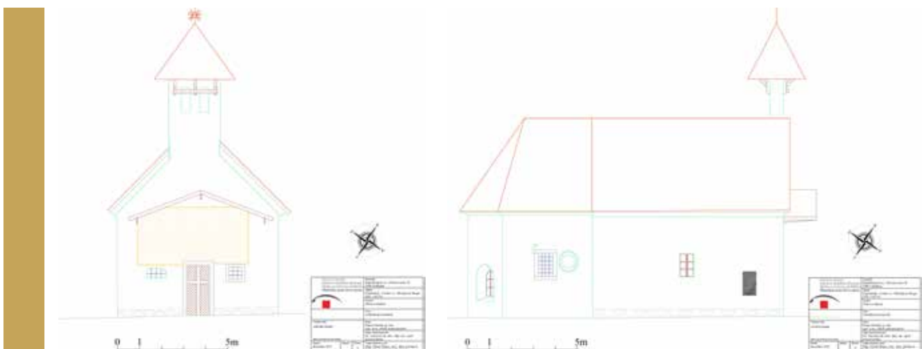
Slika 2: Pročelje (severozahodna fasada) cerkve sv. Nikolaja v Žužemberku, izdelal: Bojan Zaletelj.
