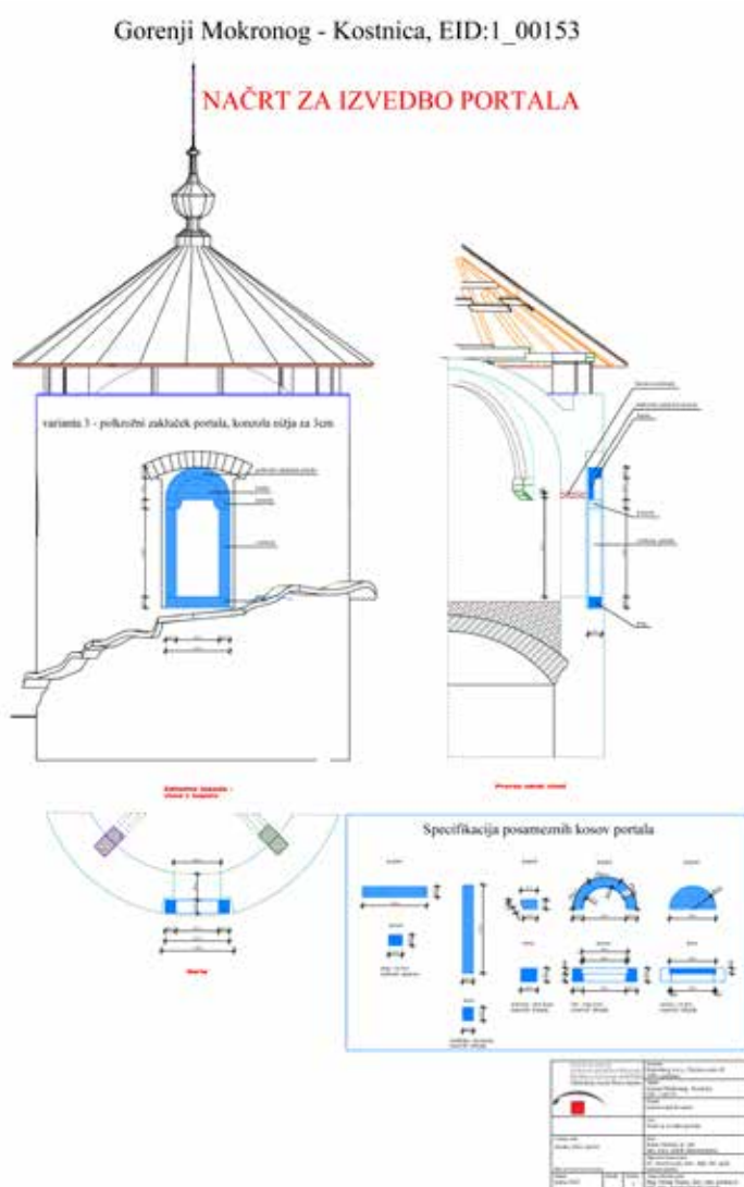
Slika 1: Načrt za izvedbo novega kamnitega portala kostnice v Gorenjem Mokronogu, izdelal: Bojan Zaletelj.
