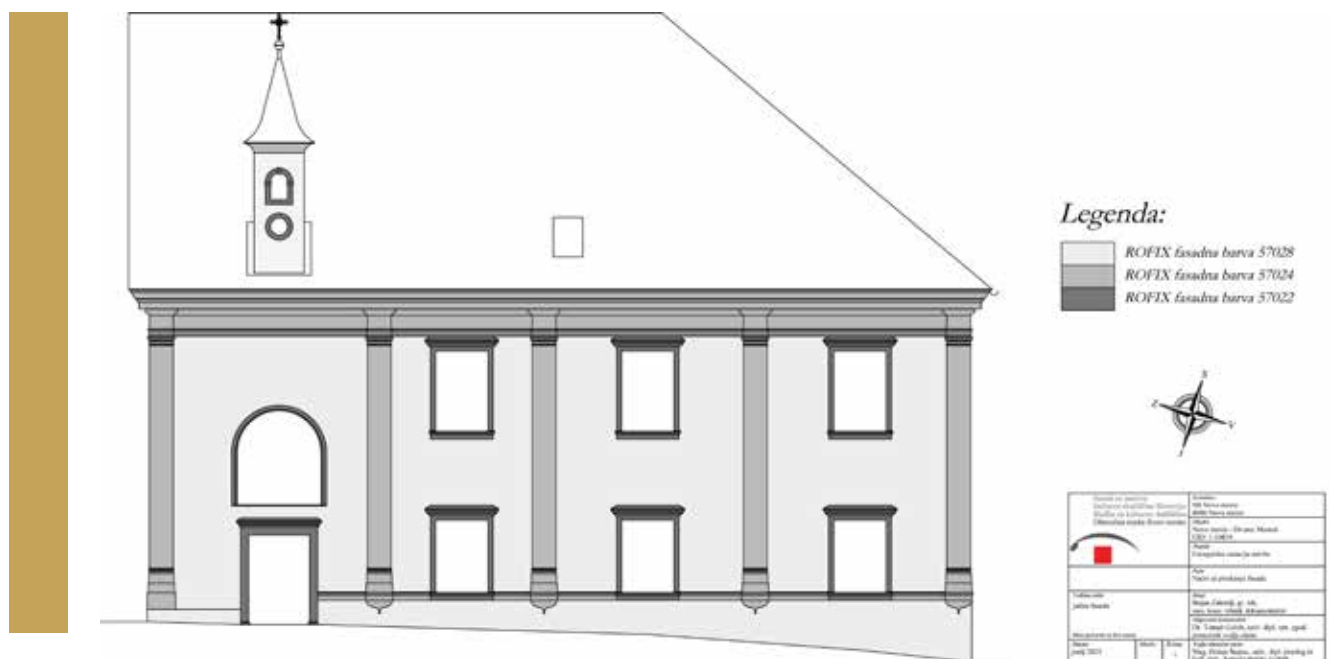
Slika 1: Barvna študija za izvedbo fasade na dvorcu Mostek v Novem mestu, izdelal: Bojan Zaletelj.
