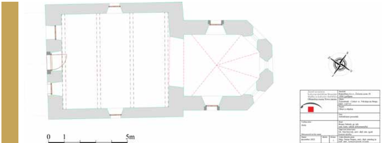
Slika 1: Tloris cerkve sv. Nikolaja v Žužemberku, izdelal: Bojan Zaletelj.
