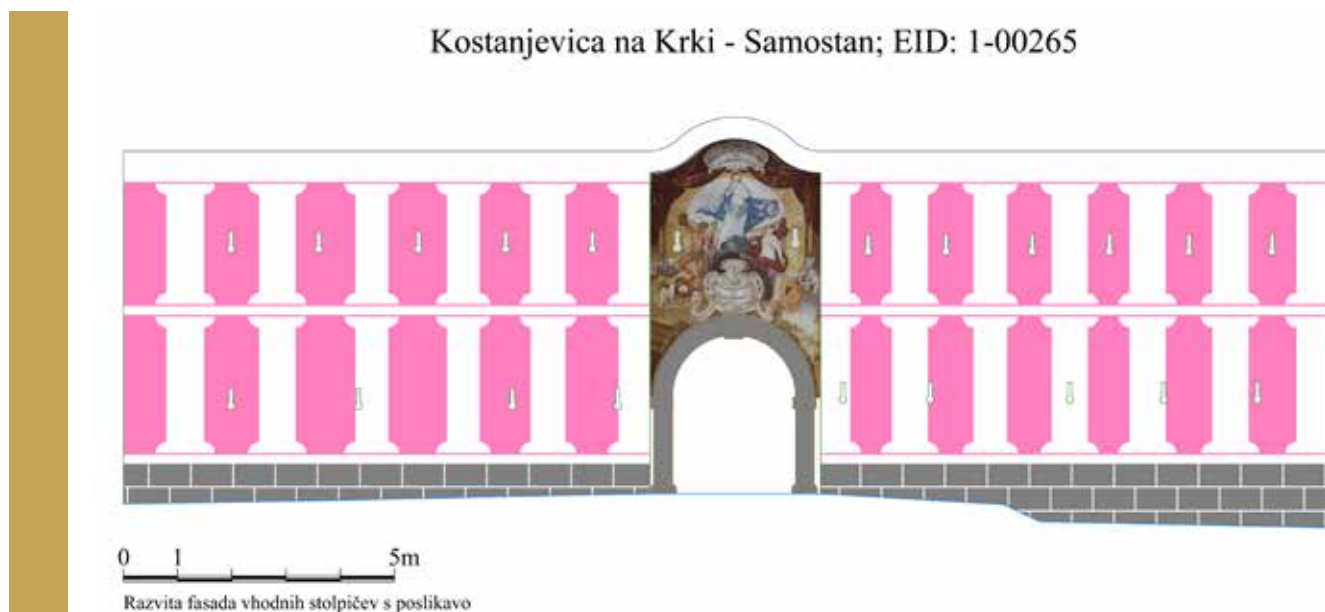
Slika 1: Razvita fasada vhodnih stolpičev s poslikavo, izdelal: Bojan Zaletelj.
