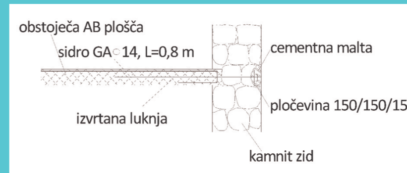
Izvedba sidranja obstoječih AB plošč • Vir: Arhiv Mojca Jarc Simonič
