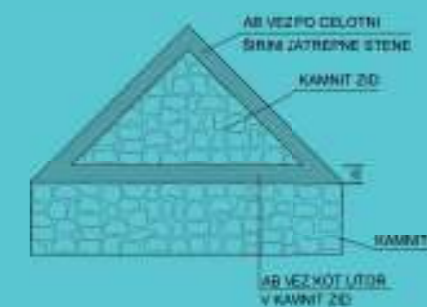
Shema utrditve zatrepne stene z vgradnjo AB vezi. Vir: Arhiv Mojca Jarc Simonič
