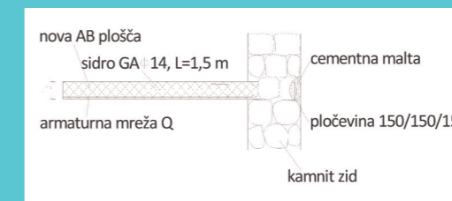
Sidranje nove AB plošče v stari zid. Vir: Arhiv Mojca Jarc Simonič
