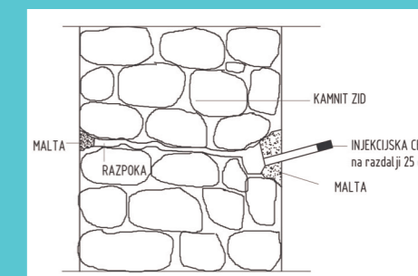
Linijsko injektiranje razpoke v kamniti steni.
