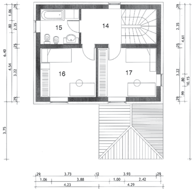
Risbe 4, 5, 6 in 7: Idejni prikaz dvonadstropne stanovanjske hiše
