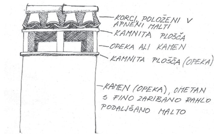
Risba 34: Navodila za obnovo dimnika
