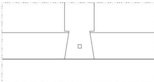
ZVEZA STEBRA IN POVEZNIKA
