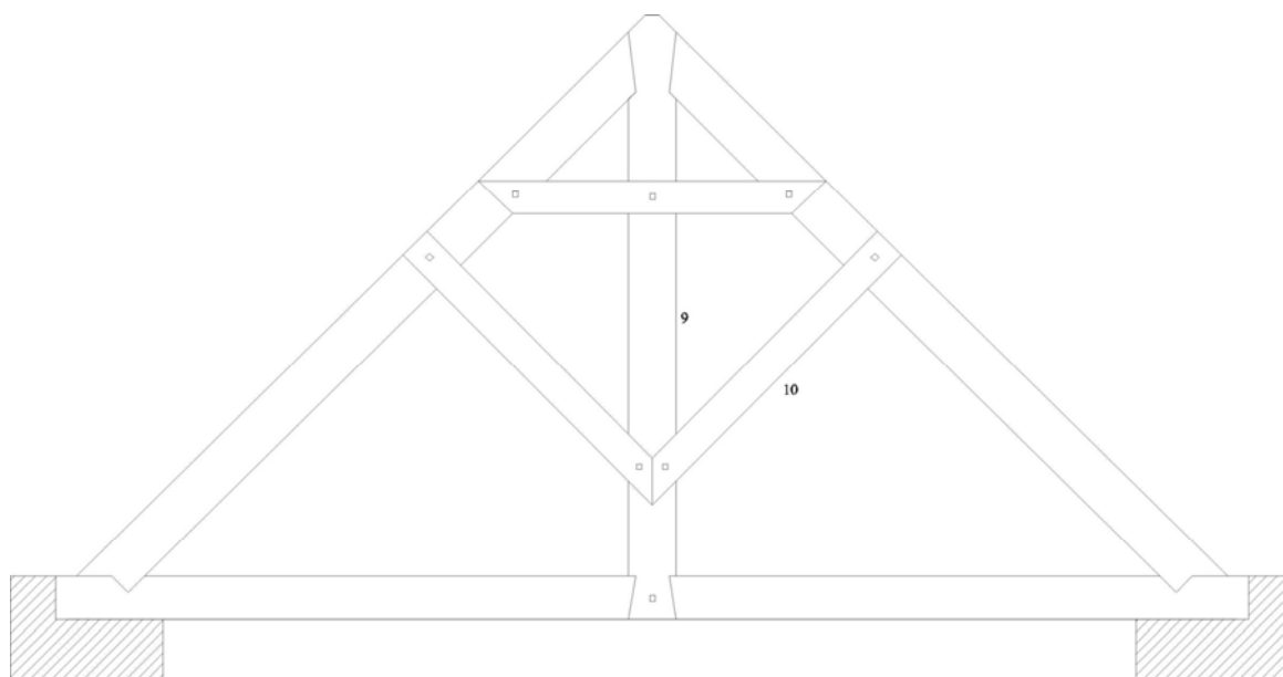
GOLTNIŠKO POVEZJE Z VRŠALOM: s (9) stebrom in z (10) ročicama
