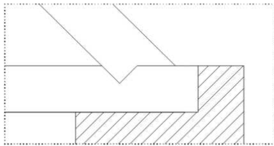
ZVEZA ŠKARNIKA S PETO IN POVEZNIKA
