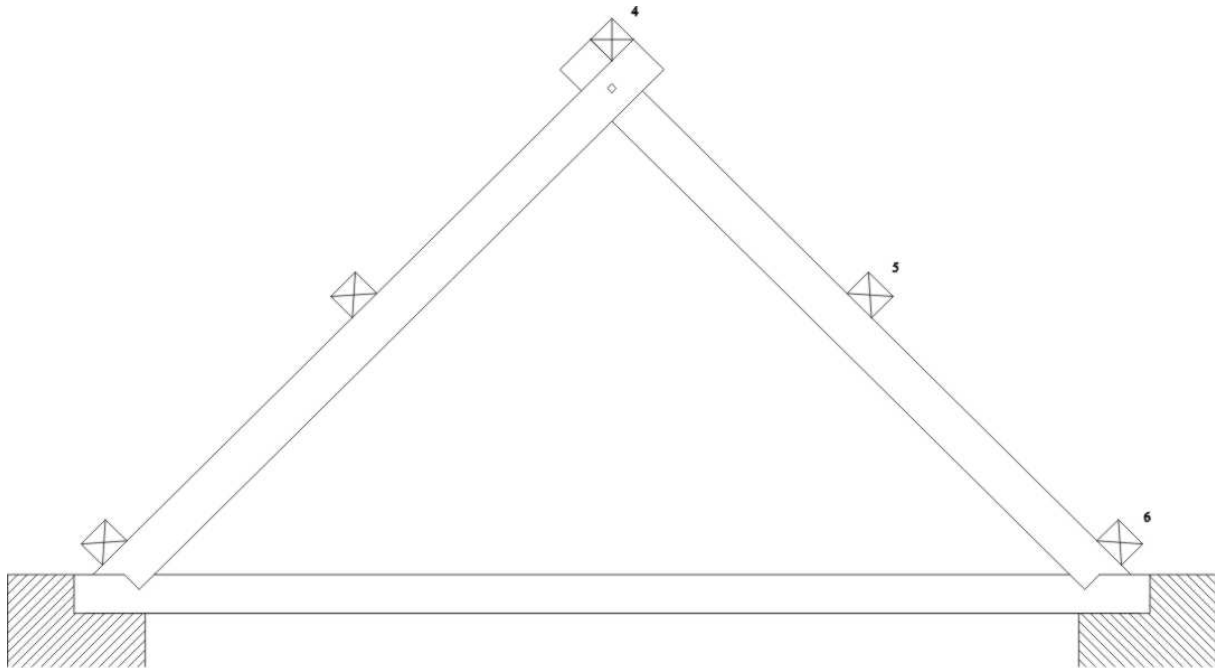
ŠKARJASTO POVEZJE Z LEGAMI NA ŠKARNIKIH: (4) slemo, (5) vmesna lega, (6) krapna lega
