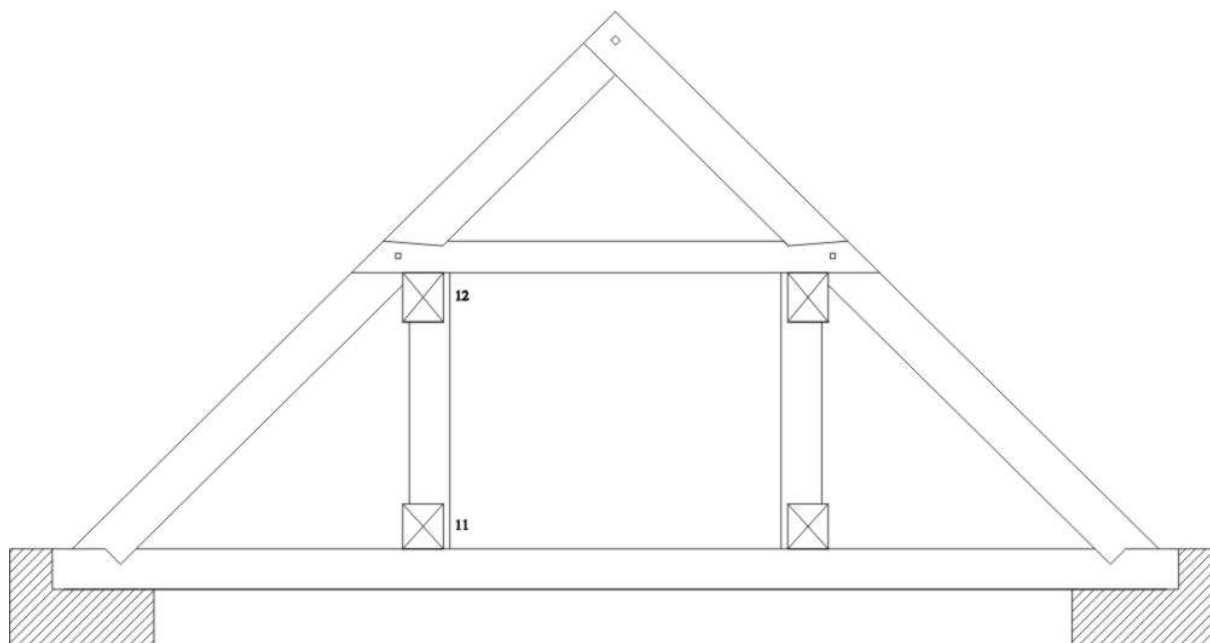
GOLTNIŠKO POVEZJE Z DVAKRAT PODPRTIM GOLTNIKOM: z vzdolžnima konstrukcijama iz (11) spodnje in (12) gornje lege ter stebrov
