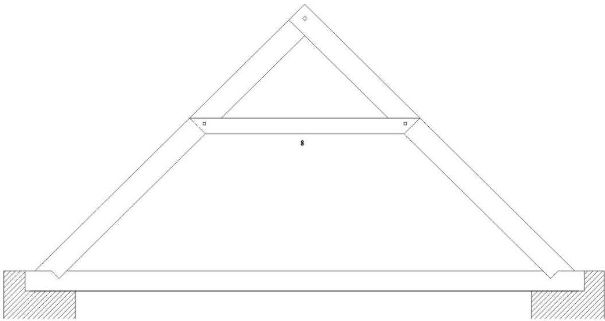
GOLTNIŠKO POVEZJE, RAZPRTO Z GOLTNIKOM (8)
