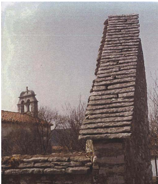
Slika 28 Na zvišanem zatrepu gospodarskega poslopja v Povirju na Krasu, ki je imelo slamnato streho, se v plasteh izmenjujejo široke (cele) in ožje (polovične) venčne skrile (foto: Franc Škrinjar, Povir, ok. 1974).
