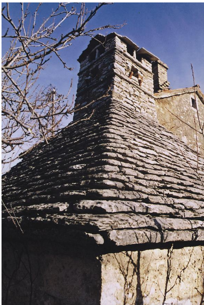
Slika 32 Grebenjaki z dvema daljšima čeloma in polovični grebenjaki z daljšim in krajšim čelom v pravokotnem grebenu šotoraste strehe na spahnjenici Kavalinovih v Povirju.
