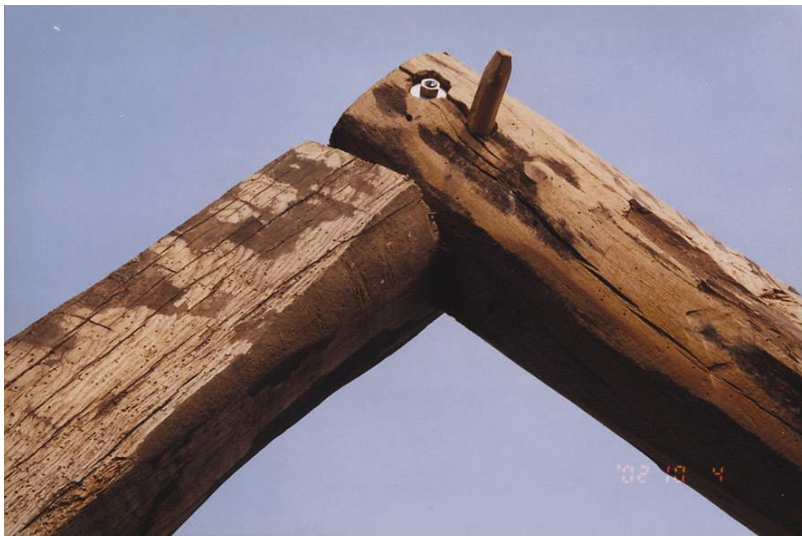
Slika 72 Detajl zveze dveh škarnikov z lesenim klinom in utopljenim kovinskim vijakom na obnovljenem ostrešju Slamčevega skednja v Pliskovici (foto Viliem Perčič, Sežana).
