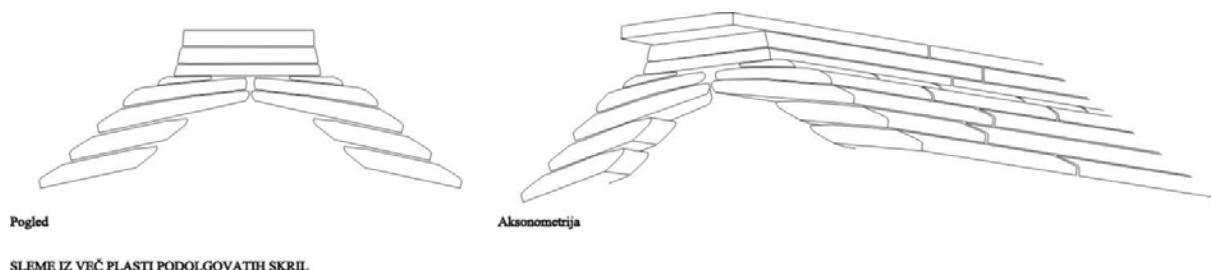
SLEME IZ VEČ PLASTI PODOLGOVATIH SKRIL
