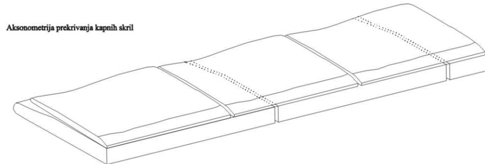
VENČNE SKRILE NA KAPU V DVEH PLASTEH (spodnje debele, zgornje tanke)
