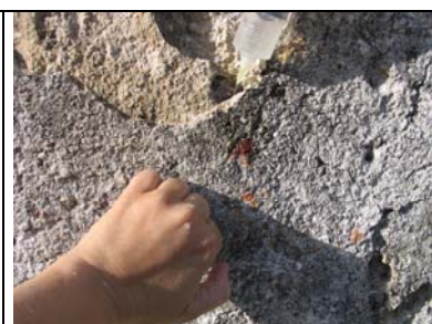
S pretrkavanjem ugotovimo votla mesta
