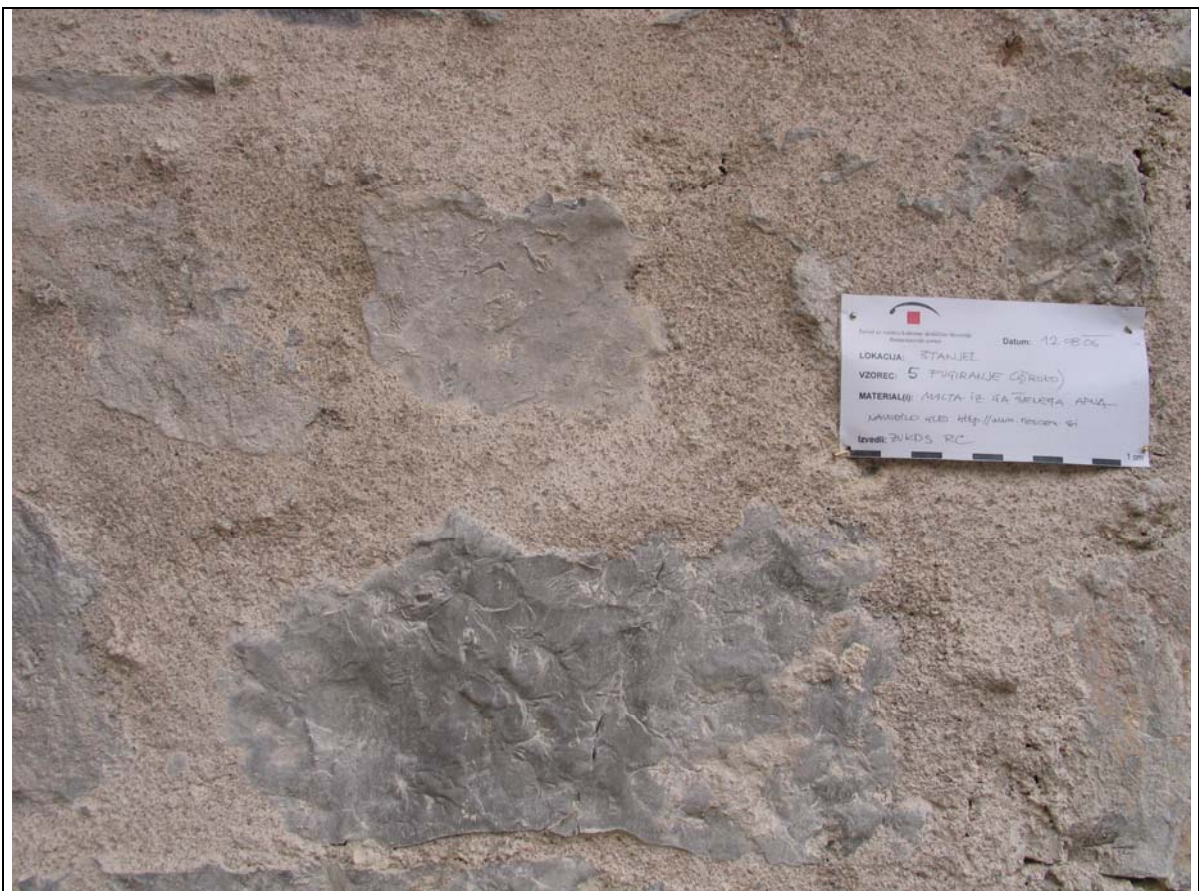
Vzorec izvedbe na hiši Markočič, Štanjel, 2006
