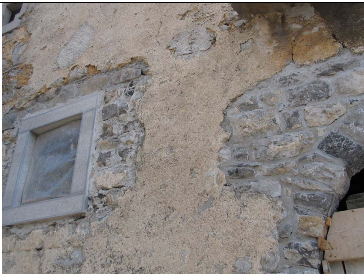
Primer ometa na fasadi hiše Lemut v Štanjelu, 2006
