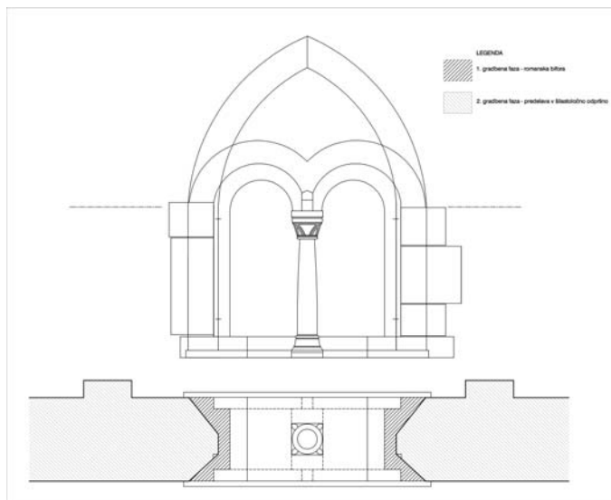
Študija predelave bifore v šilastoločno okno in najdbe romanskih kapitelov, stebričev in baz
