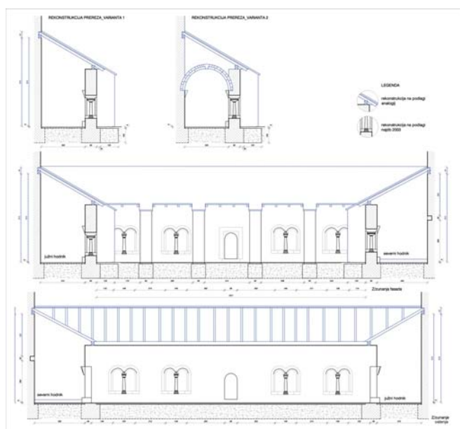
Rekonstrukcija romanske zasnove križnega hodnika in severna fasada z vidno linijo prvotne etaže križnega hodnika ter opečnih polnil ( na mestih odstranjenih opornikov) med okni.
